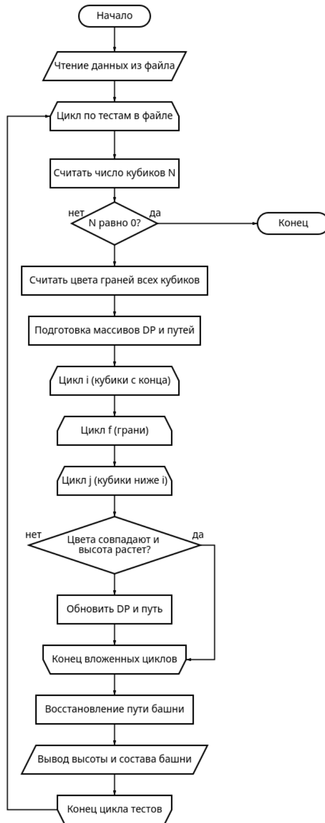
Рисунок 1 - Схема алгоритма.
